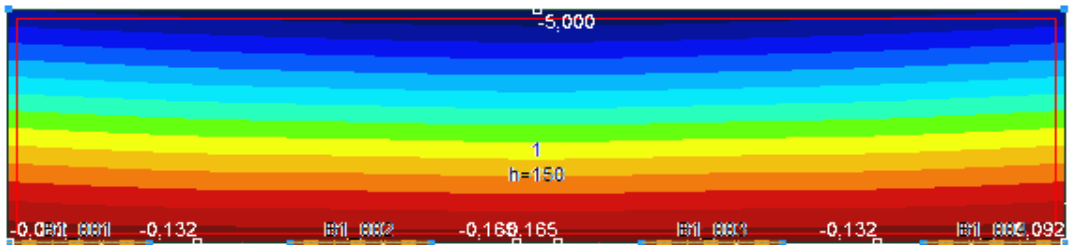
Lehajlás - SLS Kvázi-állandó - Ec,eff
