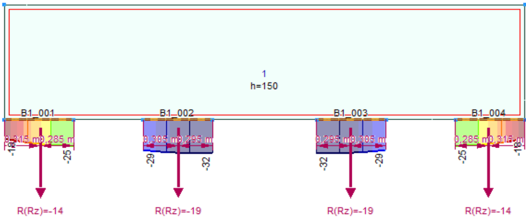
Vonalmenti támaszerő - Nyírás - ULS (a,b)
