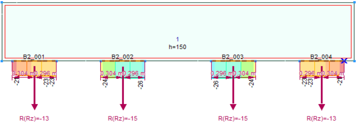
Vonalmenti támaszerő - Nyírás - ULS (a,b)
