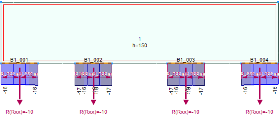
Vonalmenti támaszerő - Nyomaték - ULS (a,b)
