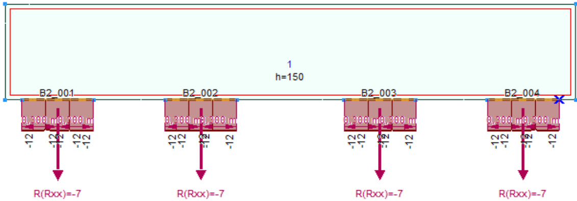
Vonalmenti támaszerő - Nyomaték - ULS (a,b)
