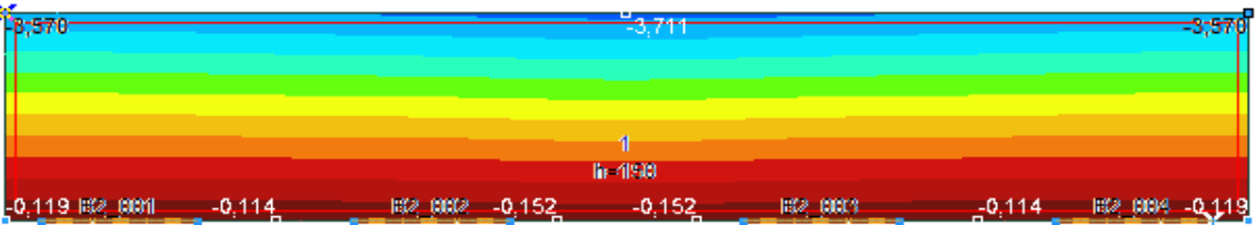
Lehajlás - SLS Kvázi-állandó - Ec,eff
